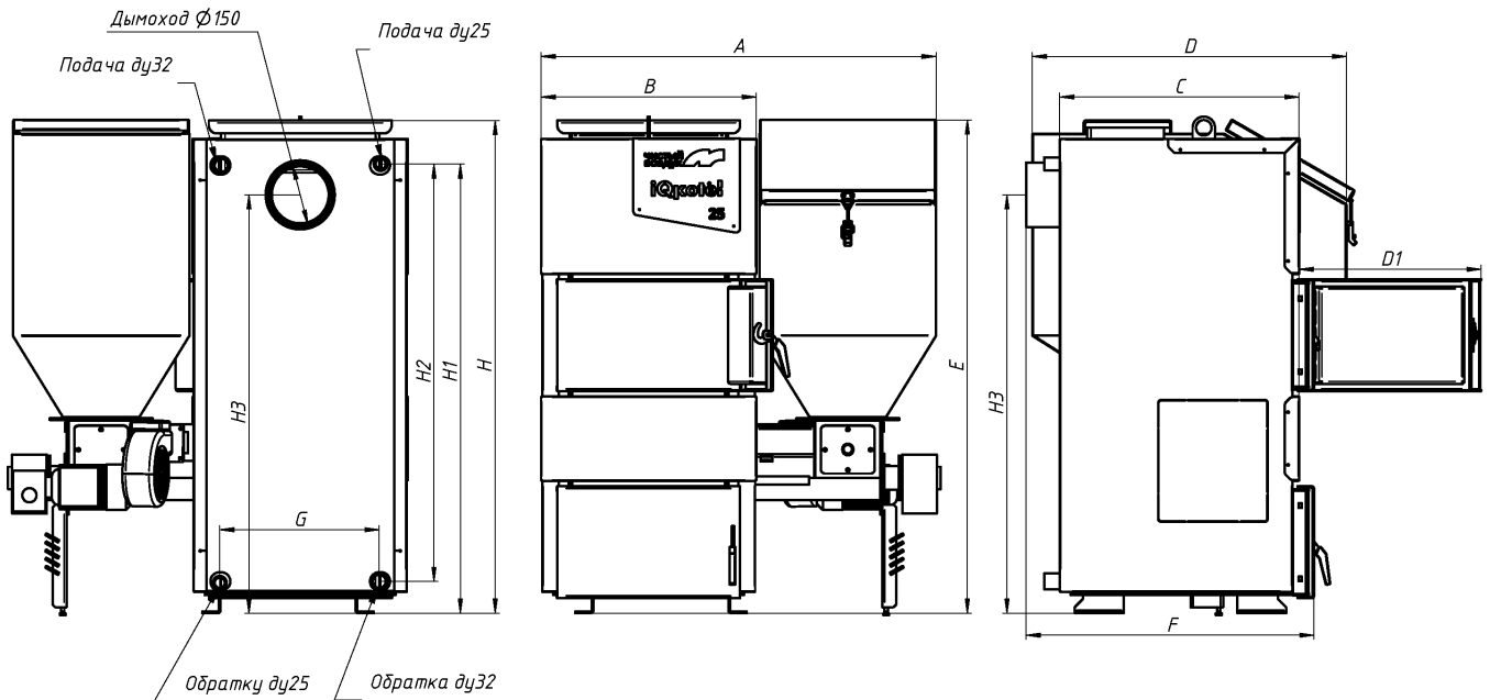
Размеры установочные (мм.) Таблица №2
