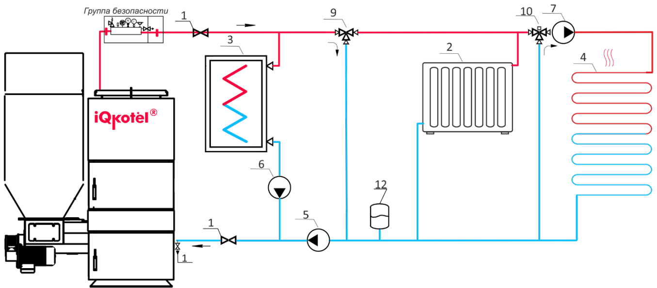
Рис. 1. Упрощенная схема подключения iQkotel Eco+ с термостатическим клапаном: iQkotel Eco+, Группа безопасности
