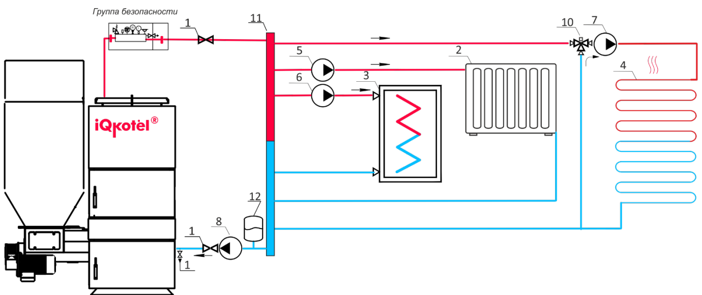
Рис. 2. Упрощенная схема подключения iQkotel Eco+ с гидравлическим разделителем: iQkotel Eco+, Группа безопасности
